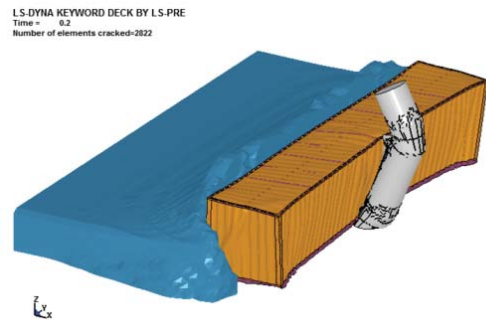
LS-DYNAを用いた漂流コンテナによるコンクリート柱の破壊挙動の解析例
