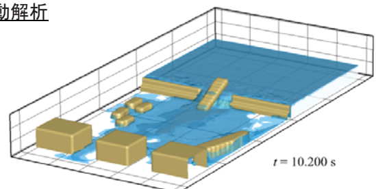
DOLPHIN-3Dによる複数の漂流物の挙動の解析例
