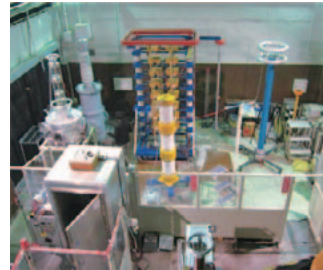
800kV 雷インパルス電圧発生装置 800kV Lightning Impulse Voltage Generator
