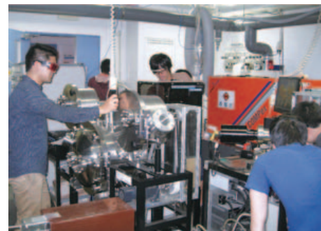
超伝導マグネットに向けた超伝導線作製装置 Fabrication system of superconducting coated conductors for superconducting magnets
