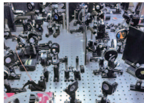
世界最高輝度のテラヘルツ波発生装置 The world highest THz wave generation system
