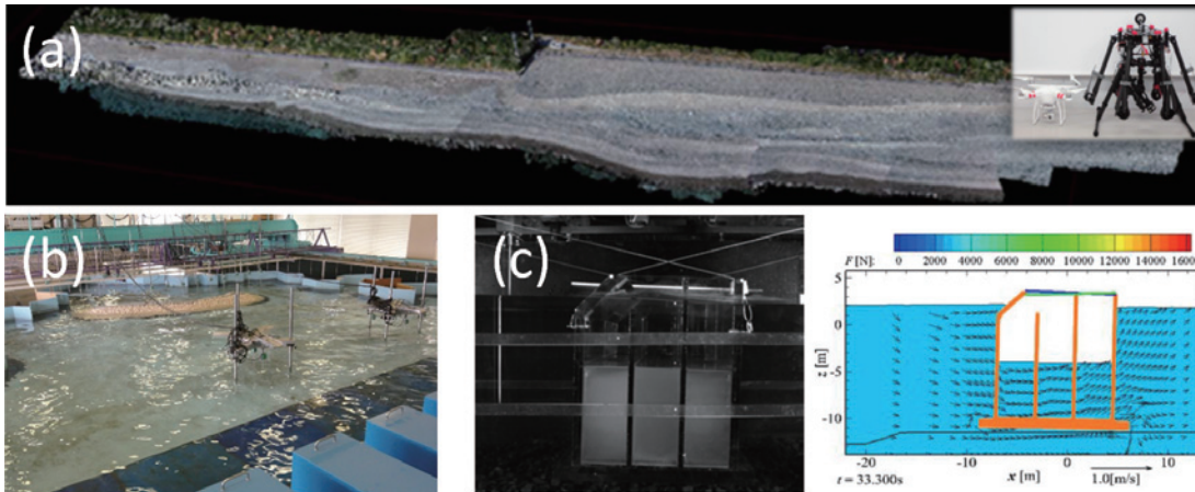
(a) UAV による地形変化観測システム (b) 高波浪時における港湾内の静穏度評価 (c) 据付作業時の防波堤ケーソンの安定性
