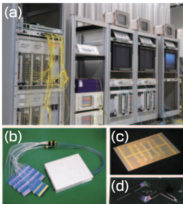
(a) 次世代光ノードシステムプロトタイプ (b) 光スイッチモジュール (c, d) 各種光集積回路チップ (a) Next generation photonic node system prototype (b) Optical switch module (c, d) Optical integrated circuit chips
